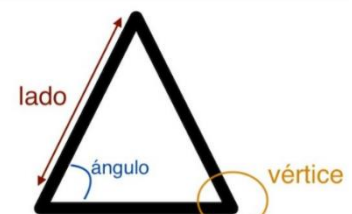
Elementos del triángulo
